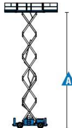
Wymiary GS-3390;GS-4390;GS-5390RT
